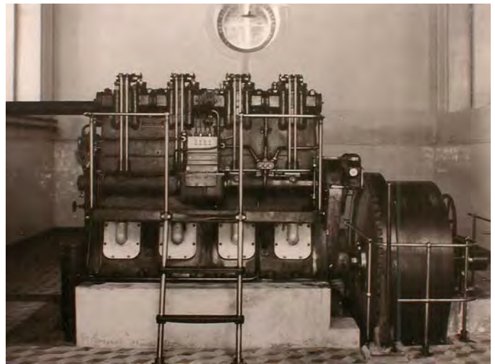
Fig. 50 – Central de produção de energia eléctrica de 1929 a partir de um motor Diesel WINTERTHUR. Foto antiga, arquivo CMO. Reprodução fotográfica de J. L. Cardoso.
