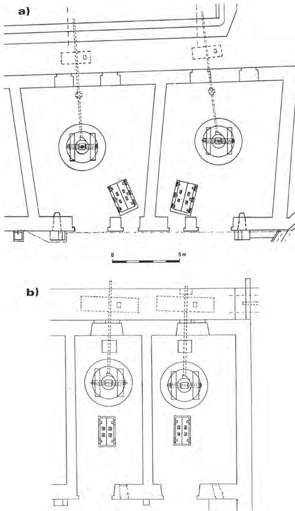
Fig. 45 – Plantas da “Fábrica de Cima” (a) e da “Fábrica de Baixo” (b), extraídas da planta geral da Fábrica de 1910, com a representação das galgas existentes em ambas, nas duas oficinas do lado setentrional, nessa época ainda em funcionamento em ambas as fábricas. Note-se o desvio do veio do engenho instalado na oficina mais setentrional da “Fábrica de Cima”, evidenciando o aproveitamento integral do comprimento do canal pré-existente do tempo das “Ferrarias” (seg. QUINTELA et al., 1995, Fig. 29).
