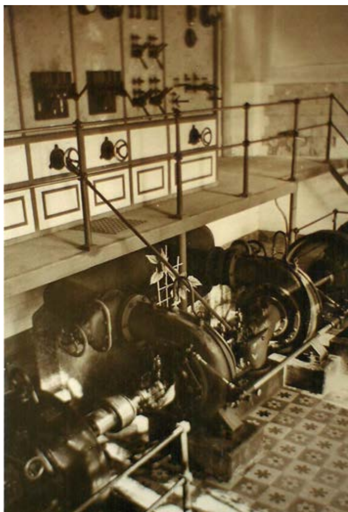
Fig. 48 – Central de produção de energia hidroeléctrica de 1925. Foto antiga, arquivo CMO. Reprodução fotográfica de J. L. Cardoso.
