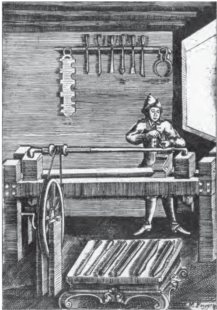
Fig. 83 – Gravura do interior de uma oficina de espingardeiro portuguesa do século XVII, com a execução da rectificação do cano da arma de fogo no engenho de verrumar, semelhante à que teria existido nas Ferrarias del Rey em Barcarena. Da obra “Espingarda perfeyta” de Cesar Fiosconi e Jordam Guserio, de 1718. Lisboa Occidental, na Oficina de Antonio Pedrozo Galram.
