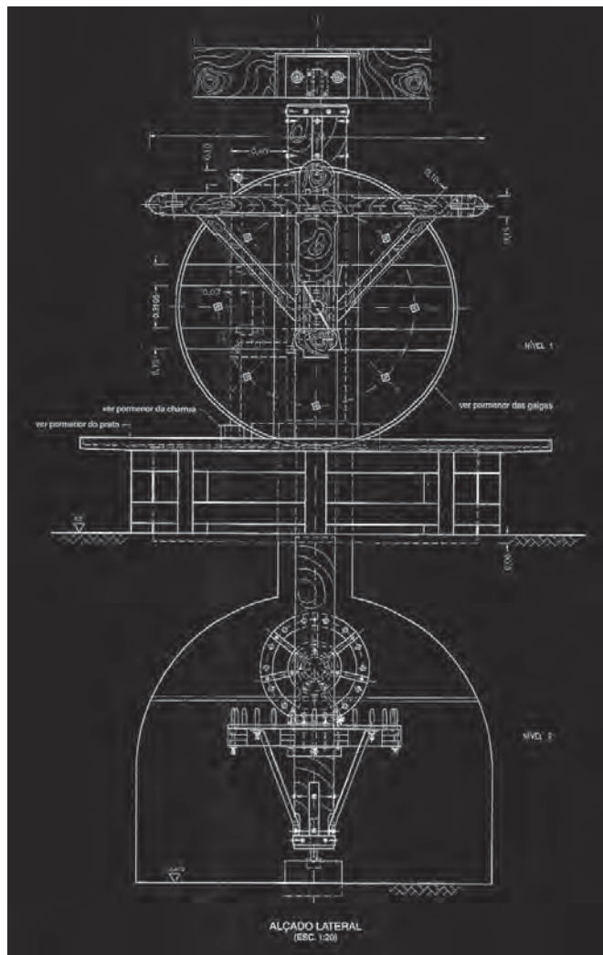
Fig. 2 – Projecto de reconstituição do sistema de galgas idealizado por Bartolomeu da Costa, utilizado na execução à escala natural do engenho exposto no Museu da Pólvora Negra. Projecto da autoria de A. Quintela, J. L. Cardoso e J. M. Mascarenhas.
